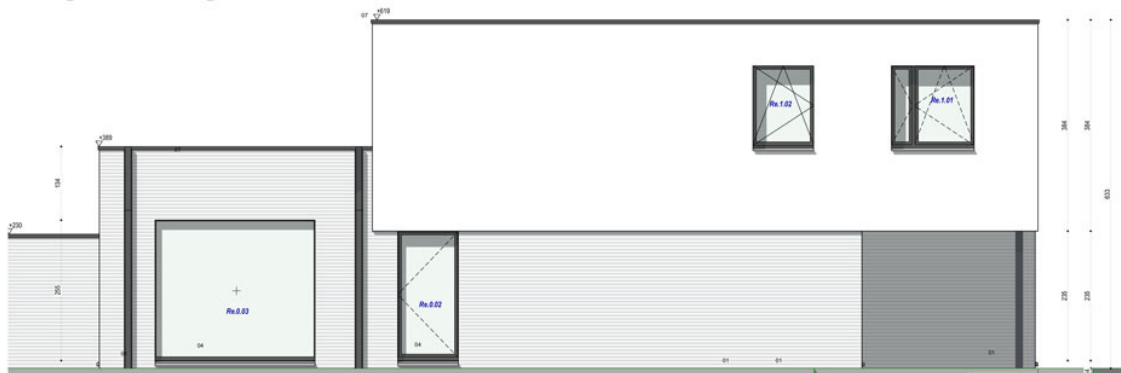
LINKERZIJGEVEL
