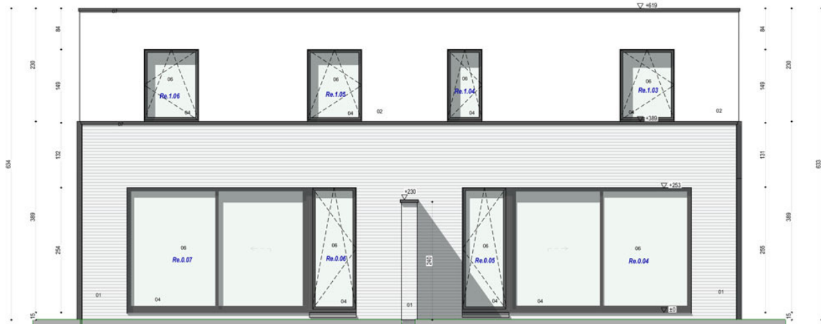
ACHTERGEVEL
